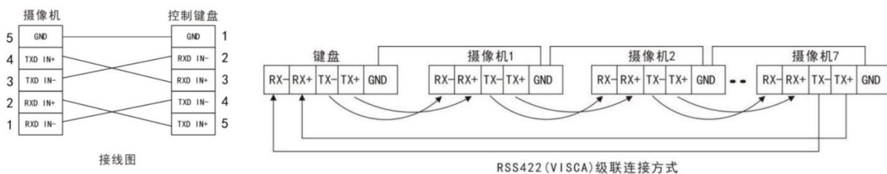
RSS422 (VISCA) 级联连接方式
