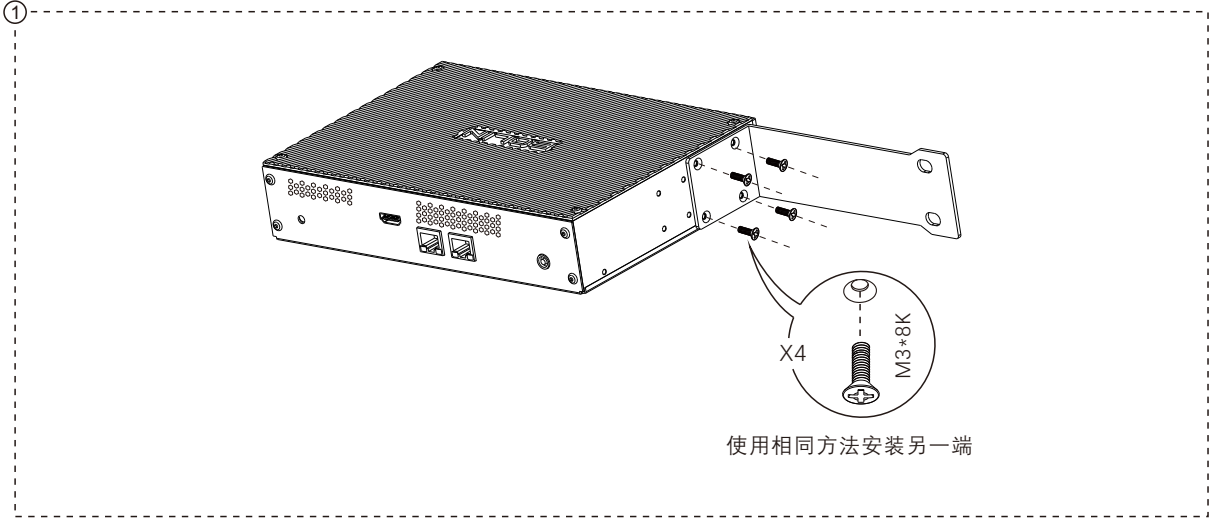
单机架安装支架 x 2
