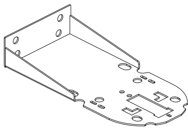
壁挂支架
